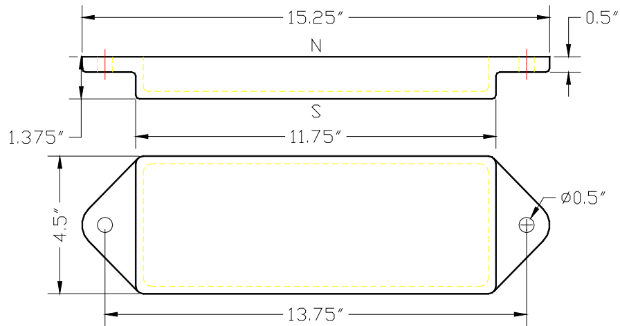
MAGNET MM-1-S
